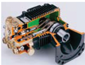
Pompe laiton en ligne avec pistons céramiques assurant robustesse et longévité
