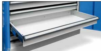
TIROIR TAILLE L LARGEUR DE L'ARMOIRE Hors tout : L. 875 x P. 450 x H.85 mm Utile : L. 845 x P. 410 x H.70 mm
