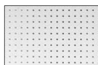
Panneau support outils en fond d'armoire Permet l'accrochage des accessoires support outils Perforations carrés 10x10 au pas de 38 mm
